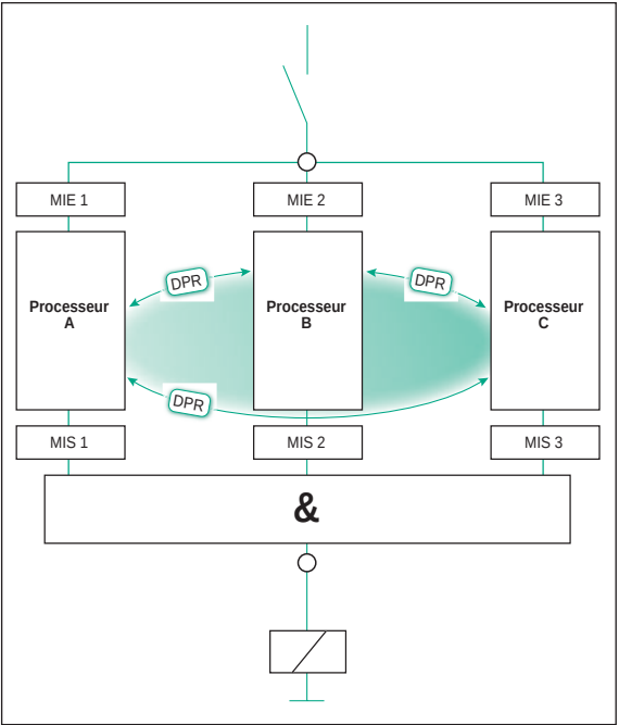
Exemple d'APIdS utilisé en commande de machines
