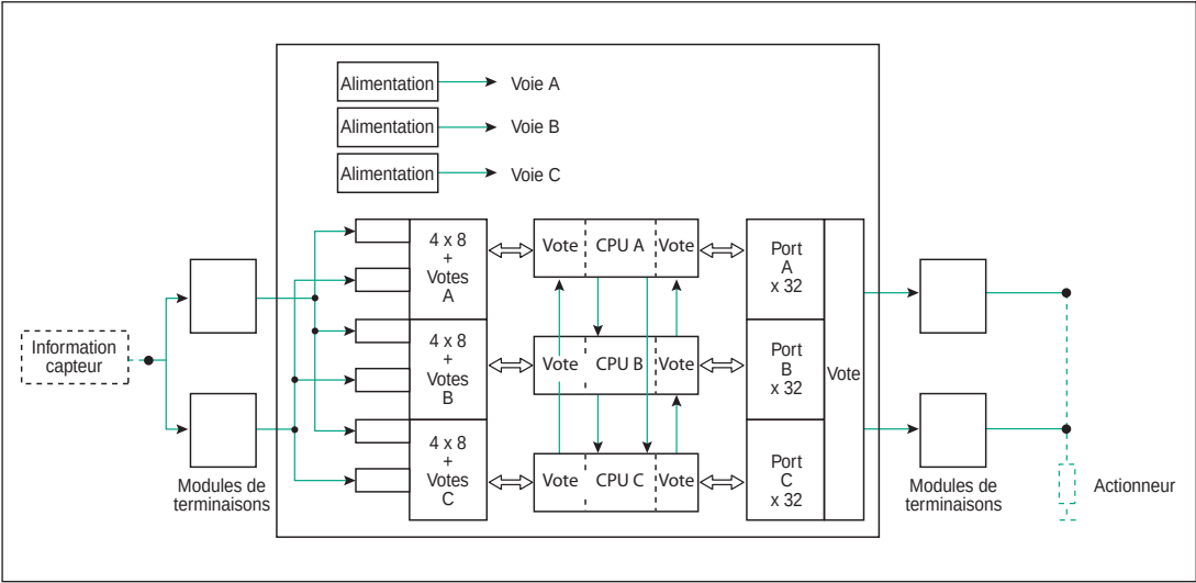
Exemple d'APIdS utilisé en commande de processus
