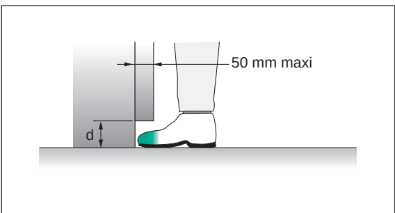
ORTEILS d mini = 50 mm
